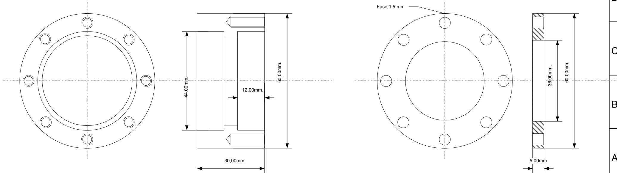
Hauptauslegerlager HL2
