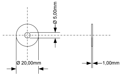
Distanzscheibe (Gummi)
