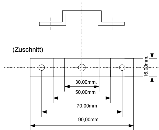
Montagewinkel
