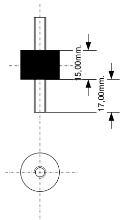
Gummidämpfer
