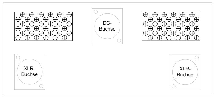
CU-CHAIN-CHASSIS Teil Lüftungsdeckel (hinten/oben) GKG1
