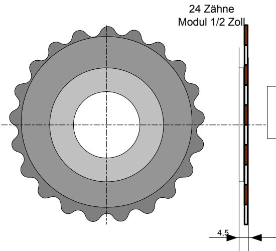
Mitnehmer-Ritzel MR1
